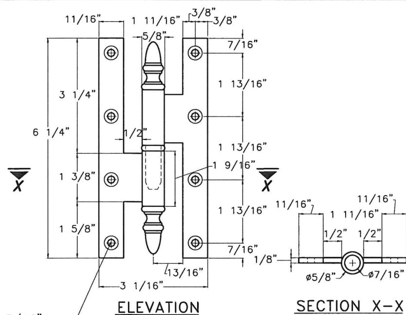
18 HINGE SCALE: 3/8" = 1"
