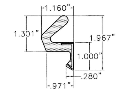
⑬ Q-LON DOOR SEAL
